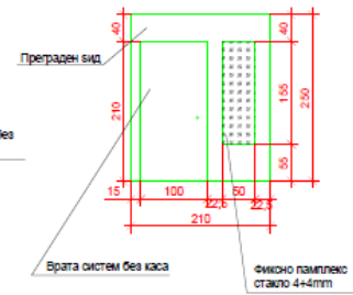
ПОЗ 6: Приемје од ходник кон трета занимална
