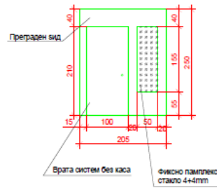
ПОЗ 5: Приемје од ходник кон прва занимална
